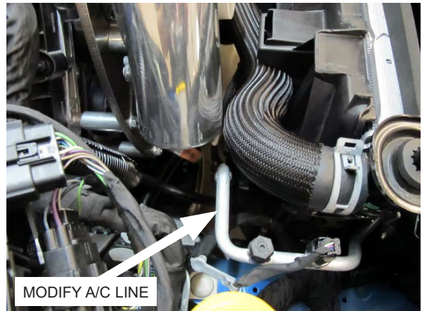
Fig. 4-af: Modify A/C Line
