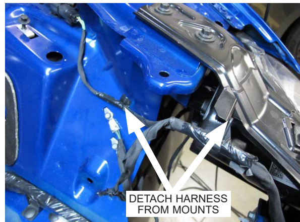
Fig. 4-al: Detach Harness
