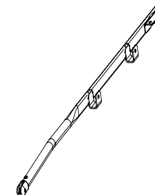
Rail latéral avant gauche Pièce n°600.83 Qté. 1
