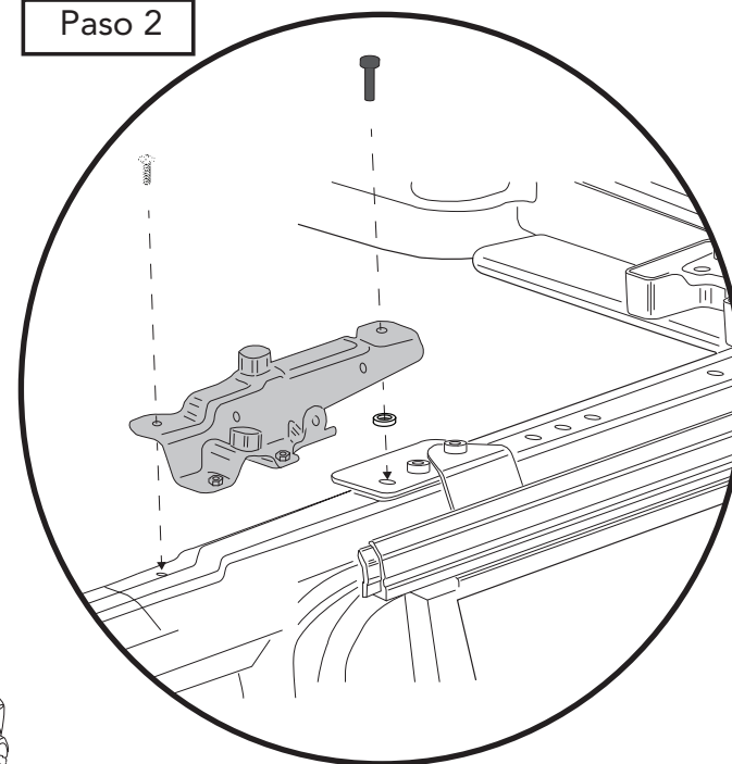
Separador, 5.5 MM Parte N° 603.20 Cant. 2
