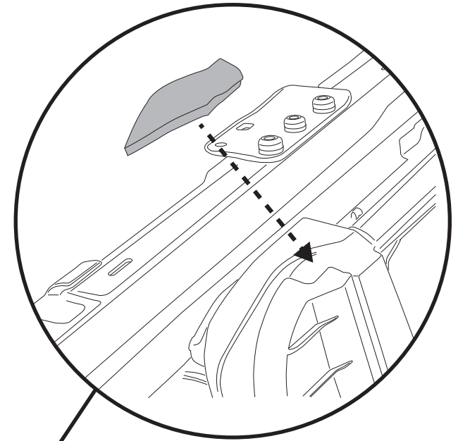
Joint de retenue verticale de fenêtre gauche Pièce n°608.73 Qté. 1
