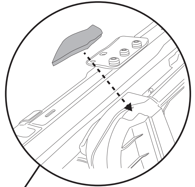
Junta de contención de la ventana vertical izquierda Parte N° 608.73 Cant. 1
