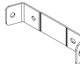
Soporte de montaje del halo trasero Parte N° 599.39 Cant. 2
